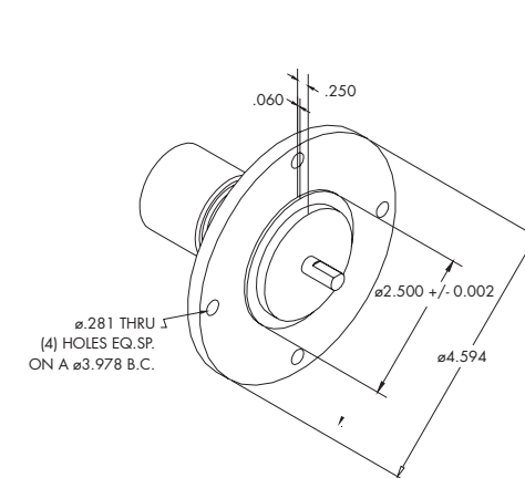
Fig. 8 DA Mount
