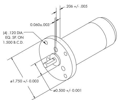
Fig. 6 SU Large Flange
